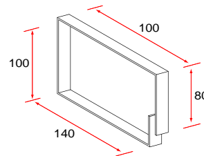
Horizontal Wire Guide
